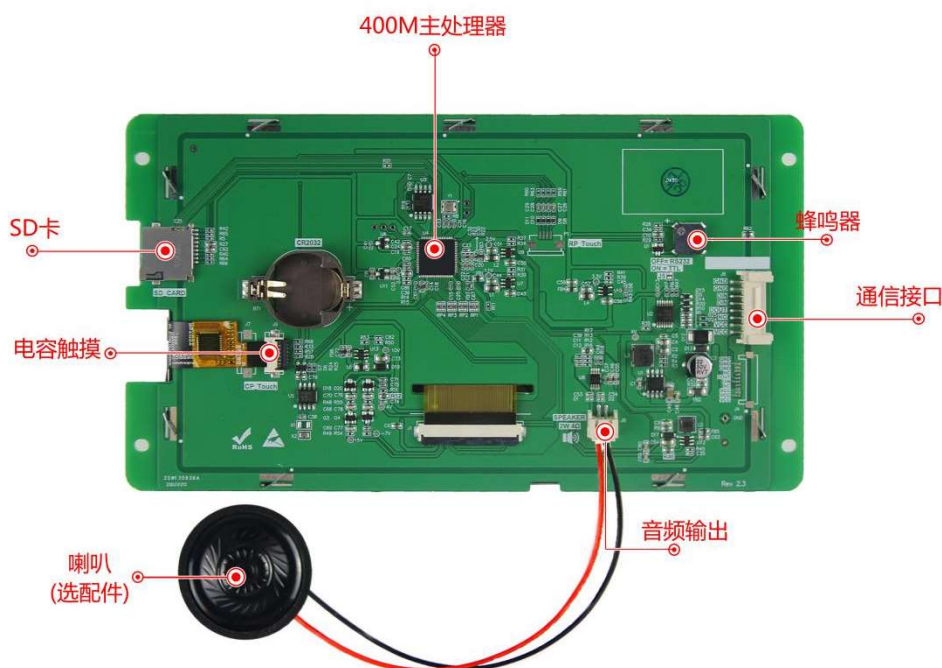
图 1-2 硬件配置图
