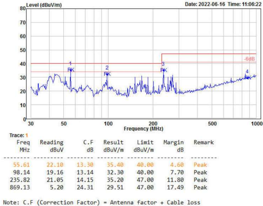
图 4-6 RE 测试垂直方向
