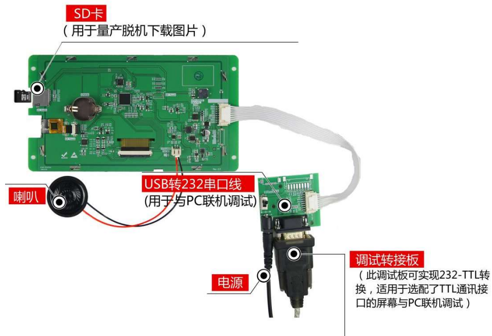
图 1-3 调试工具图
