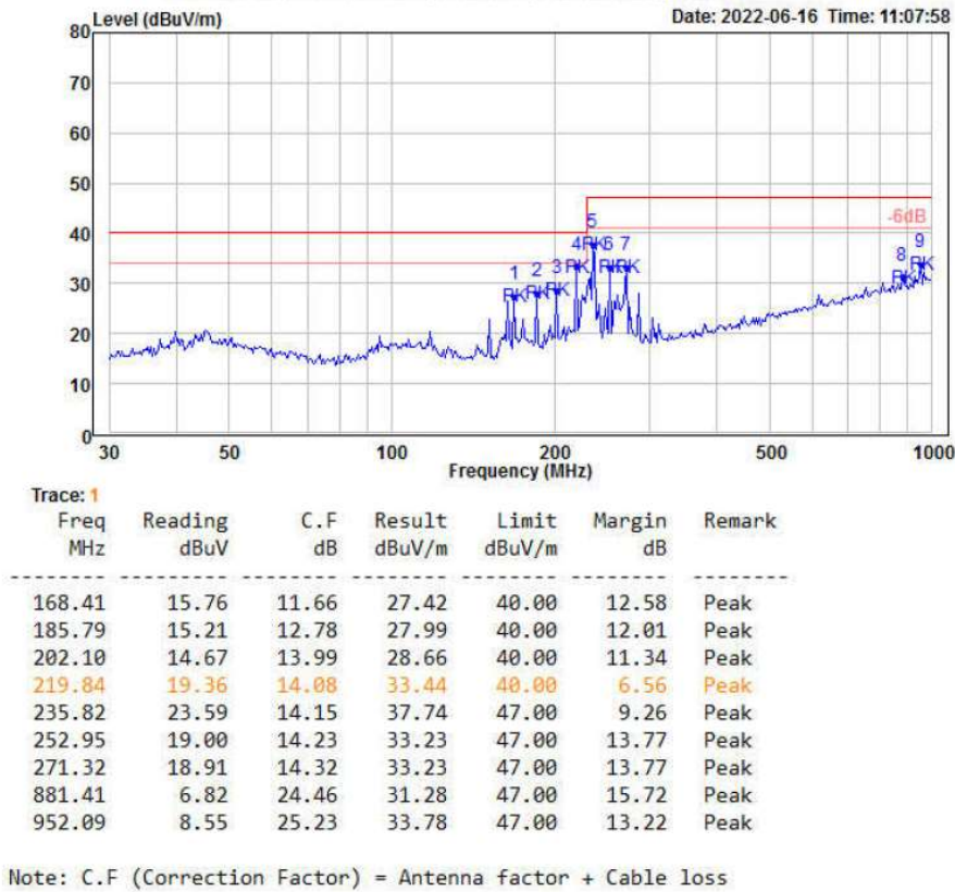
图 4-5 RE 测试水平方向
